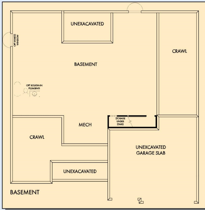
OPTIONAL BASEMENT
