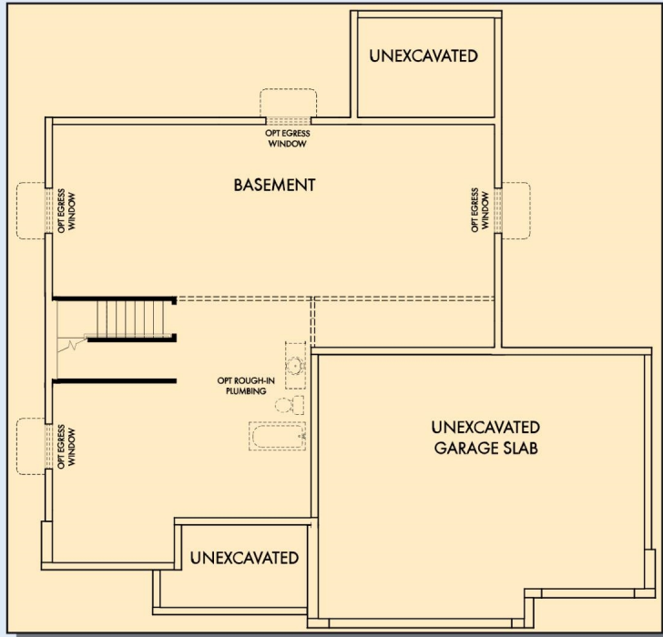
OPTIONAL BASEMENT
