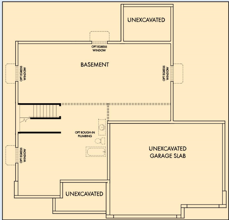
OPTIONAL BASEMENT
