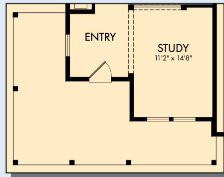
OPTIONAL WRAPPED PORCH
