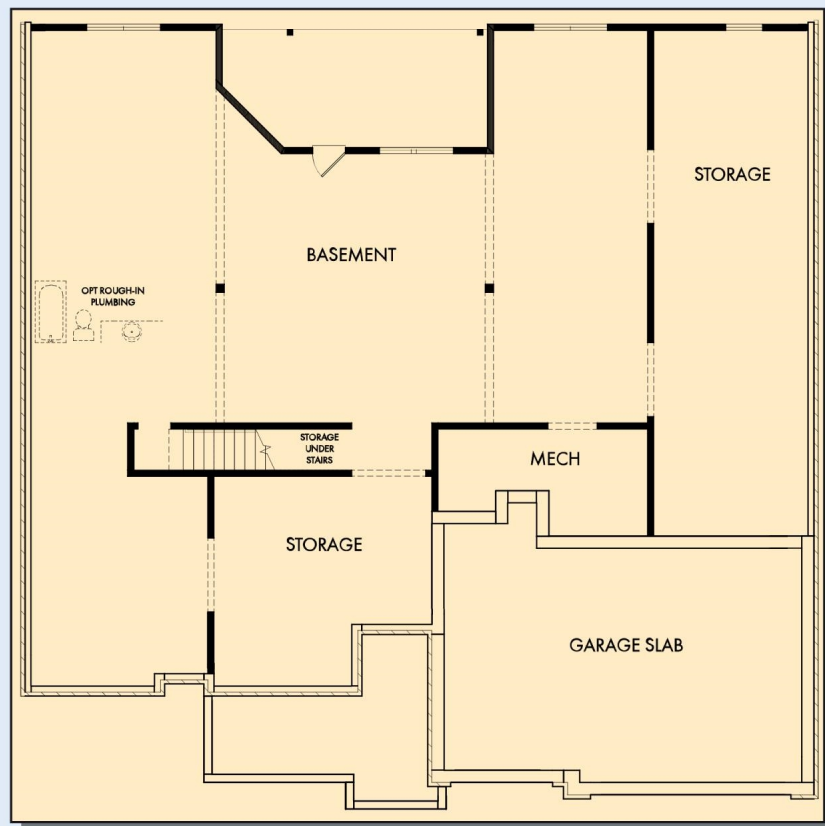
OPTIONAL BASEMENT
