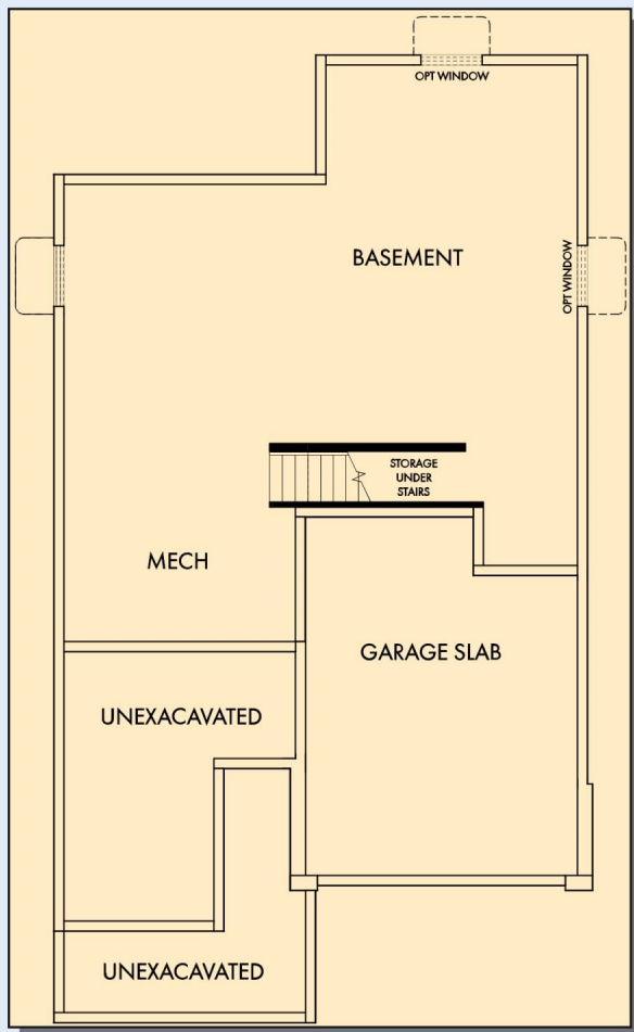
OPTIONAL BASEMENT
